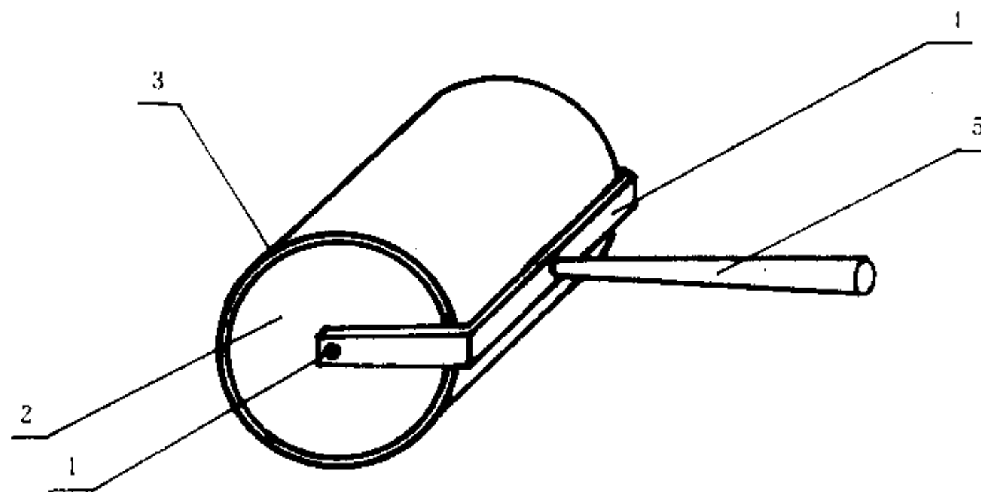
图 5 滚筒示意图
